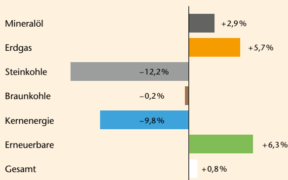
Entwicklung des Primärenergieverbrauchs in 2017 in Deutschland
