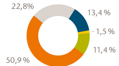
Bundesdeutscher Strommix 2)
